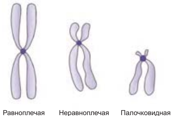
Рис. 46. Типы хромосом
