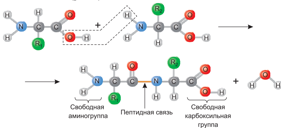
Рис. 7. Синтез дипептида
